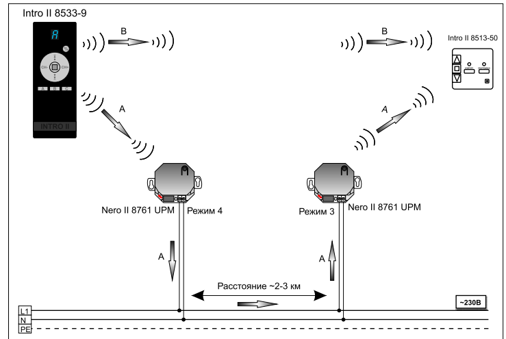
Рисунок 2 Пример реализации функции «Мост» по сети ~230 В
