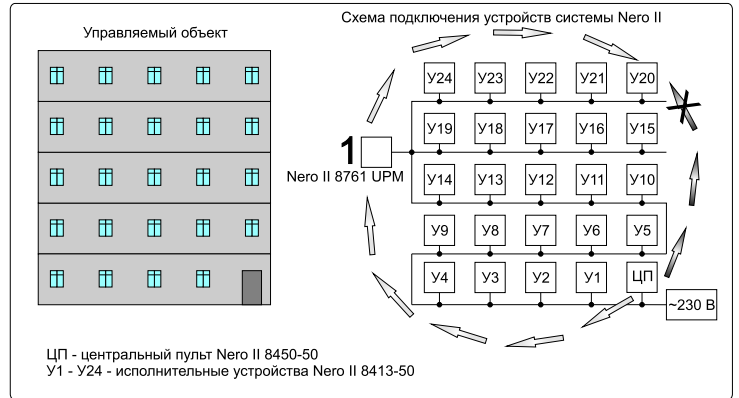
Рисунок 5 Пример реализации режима «ретранслятор» по сети ~230 В
