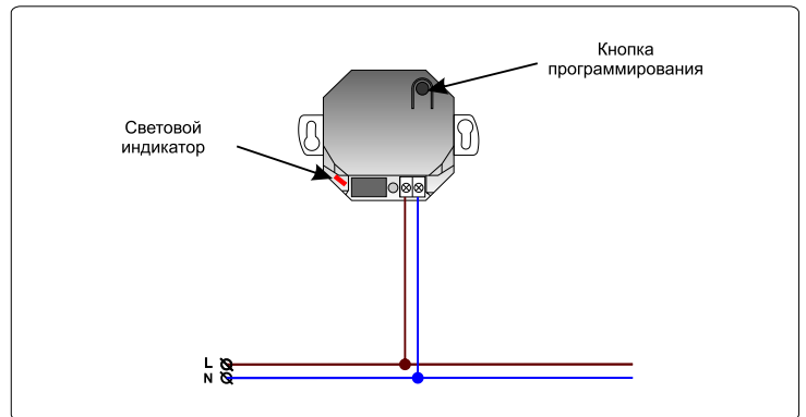
Рисунок 6 Типовая схема подключения Nero 8761 UPM
