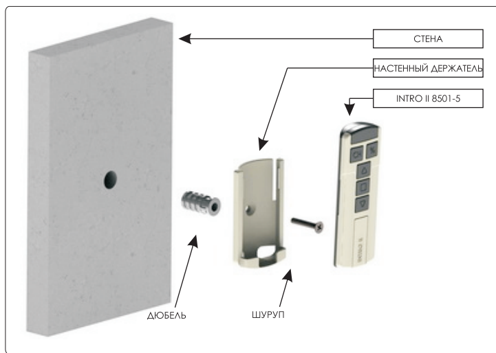
Рисунок 4 Монтаж устройства Intro II 8501-5
