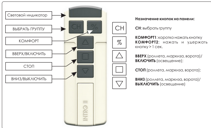
Рисунок 1 Назначение кнопок на лицевой панели Intro II 8501-5
